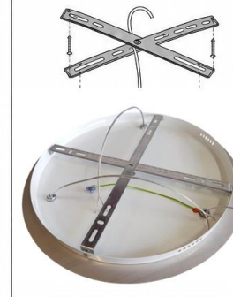
VISTA SUPERIORE ATTACCO ROSONE
