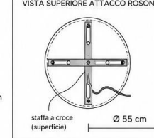
VISTA SUPERIORE ATTACCO ROSONE
